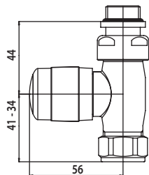
Valvola e Detentore dritti Figura 2
