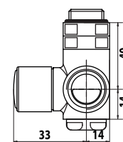
Valvola e Detentore per funz. misto Figura 6
