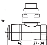
Valvola e Detentore a squadra Figura 1
