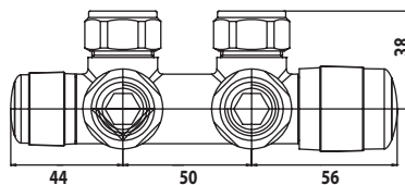
Gruppo Valvola e Detentore a squadra passo 50 mm Figura 3
