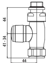
Valvola e Detentore dritti Figura 2
