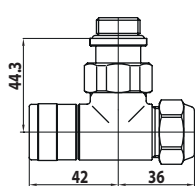
Valvola e Detentore a squadra Figura 4
