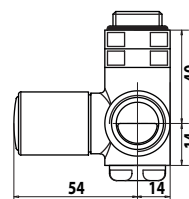
Valvola e Detentore per funz. misto Figura 6
