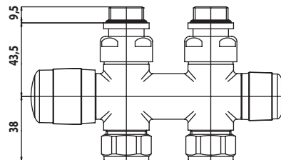
Gruppo Valvola e Detentore dritto passo 50 mm Figura 3
