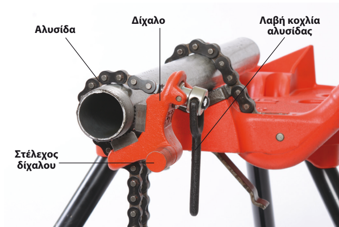
Εικόνα 6Α – Τοποθέτηση δίσκου σύνθετου σωληνοκάβουρα σε σωλήνα
