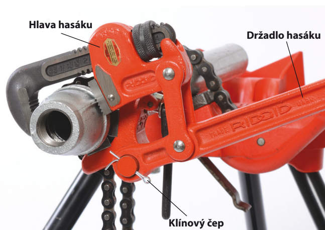
Obrázek 6B – Zajištění držadla na radiálním čepu
