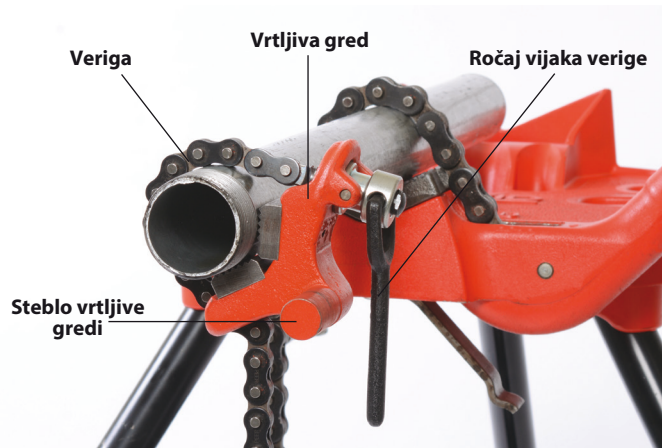
Slika 6A - Montaža vrtljive gredi ključa s sestavljenim vzvodom na cev
