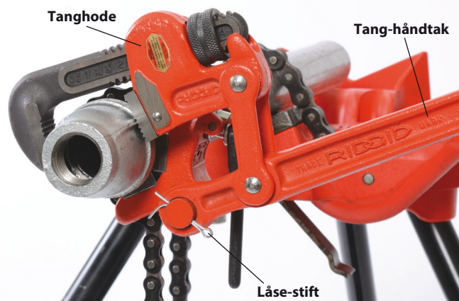
Figur 6B – Feste håndtaket til kingbolten
