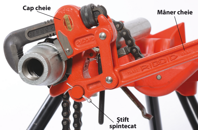
Figura 6B – Fixarea mânerului la reazemul cu fus
