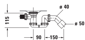
Sifone per vasca idromassaggio # 760450
