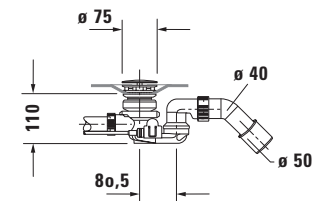
Sifone con alzata dal pavimento per vasca # 700449
