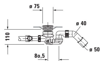
Sifone con alzata dal pavimento per vasca idromassaggio # 760450
