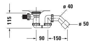
Sifone per vasca idromassaggio # 760449
