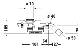
Sifone per vasca # 700450
