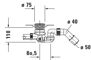
Sifone con alzata dal pavimento per vasca # 700453
