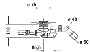
Sifone con alzata dal pavimento per vasca idromassaggio # 760449
