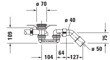
Sifone per vasca # 700449
