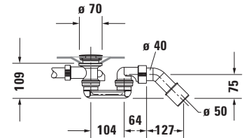
Sifone per vasca # 700453
