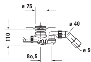
Sifone con alzata dal pavimento per vasca # 700450
