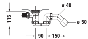
Sifone per vasca idromassaggio # 760451
