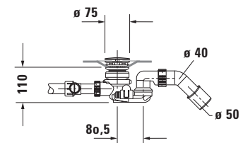
Sifone con alzata dal pavimento per vasca idromassaggio # 760451
