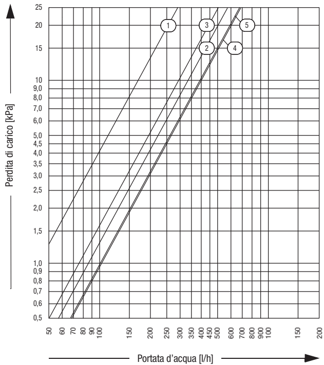
Tivano, Tivano R - Raffreddamento
