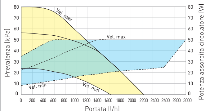
Grafico zona miscelata optional (prevalenza a velocità fissa-valvola miscelatrice aperta)
