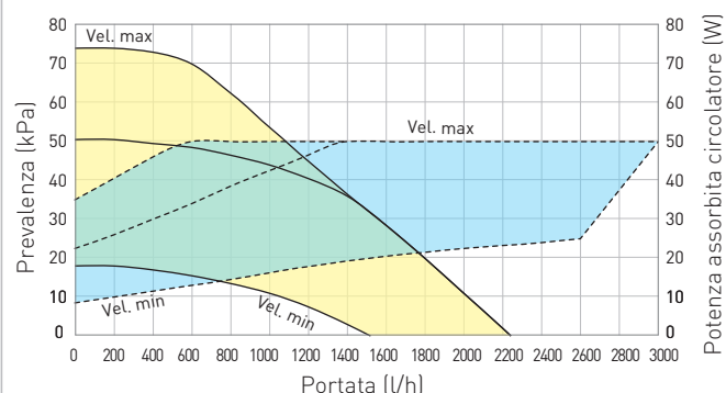
Grafico zona diretta di serie (prevalenza a velocità fissa)
